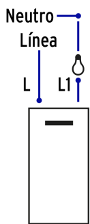
Interruptor sencillo
