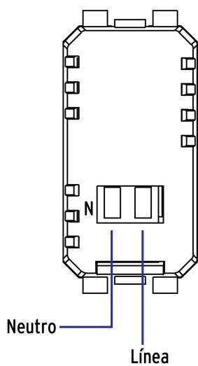
Diagrama de conexión
