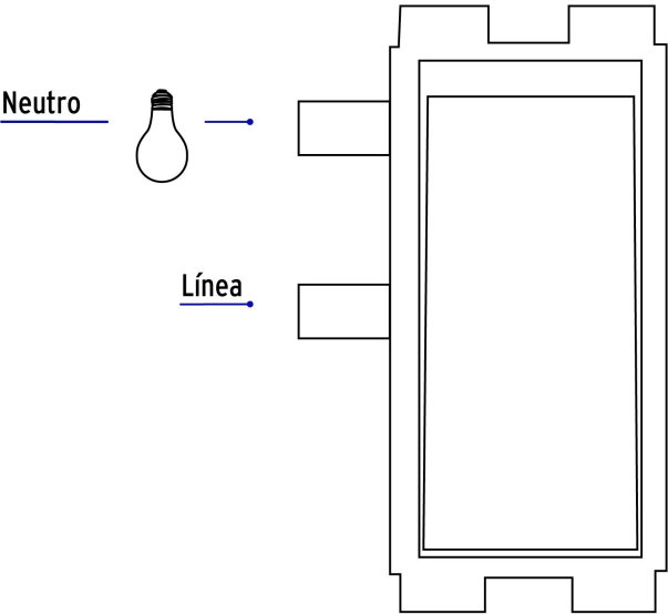
Diagrama de conexión
