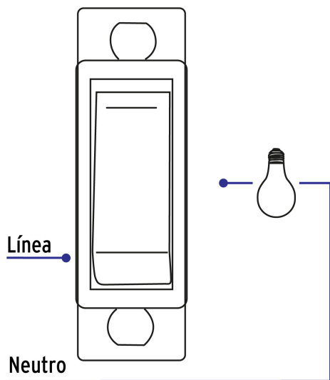
Diagrama de conexión
